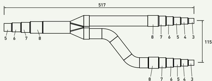
Plynové potrubí
