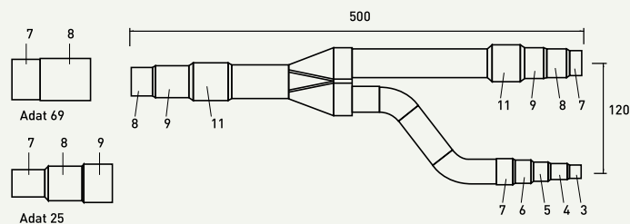
Plynové potrubí
