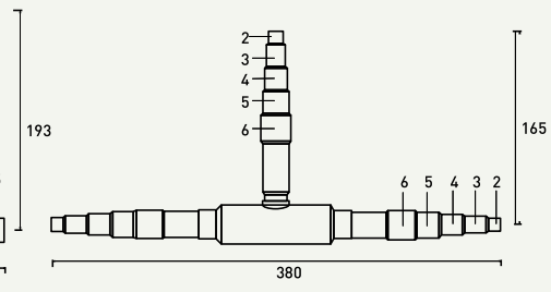
Kapalinové potrubí
